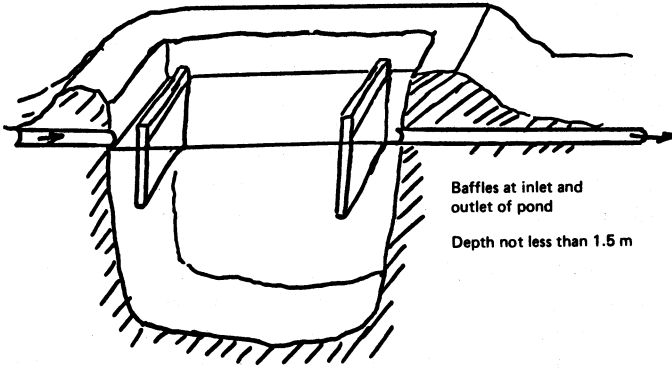
Fig. 30. ANAEROBIC STABILIZATION PONDS
