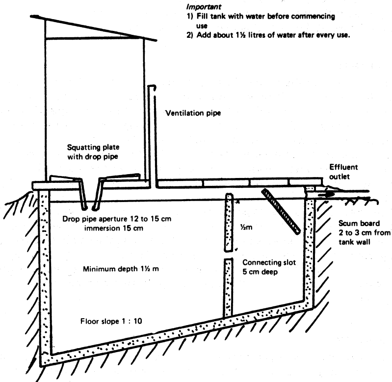
Fig. 28. THE AQUA PRIVY
