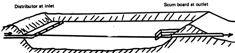
Fig. 31. AEROBIC STABILIZATION PONDS
