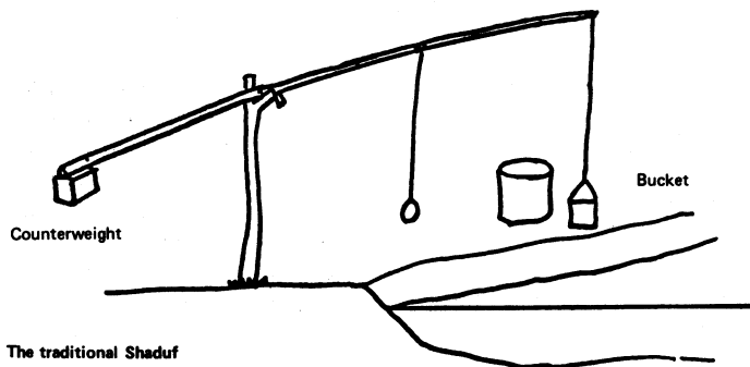
Fig. 18. THE SHADUF
