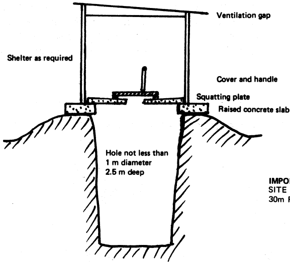
Fig. 26. THE PIT PRIVY
