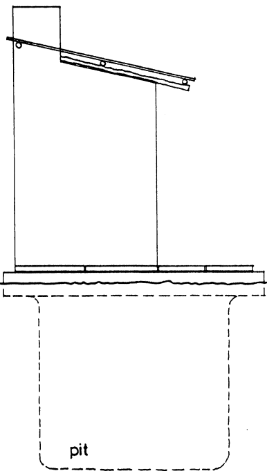
END ELEVATION
